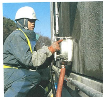
コンクリート構造物の目粗し
